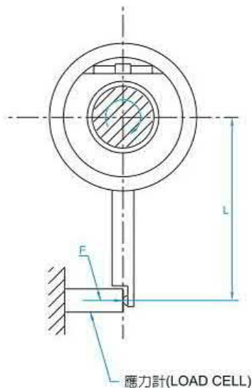
預壓動扭矩測定法
