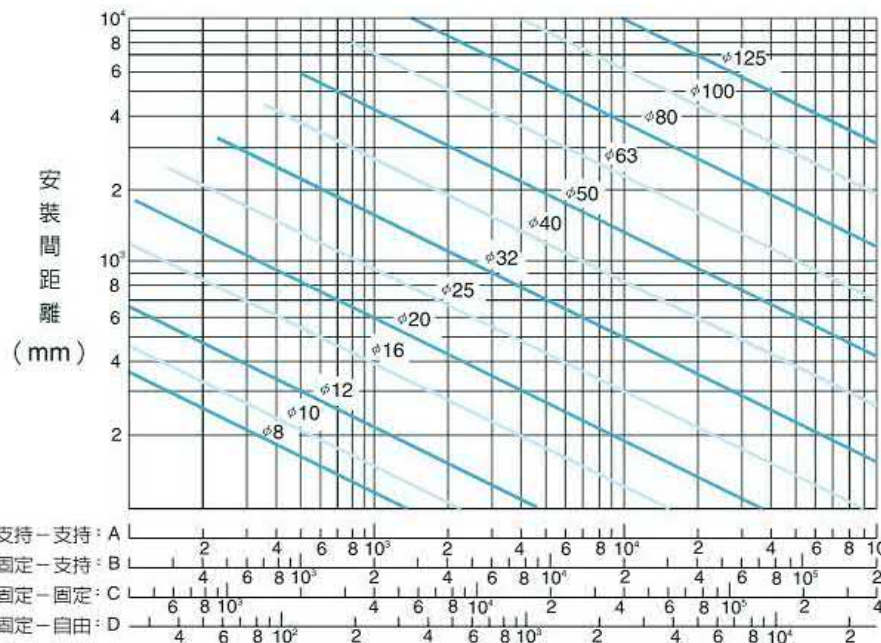
圖 4.2.2.1 挫屈之容許壓縮負荷
