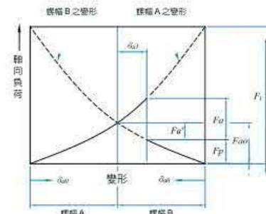
圖 4.4.1.4 定位預壓變形關係圖
