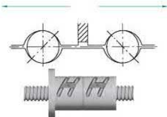
圖 4.4.1.1 伸張預壓
