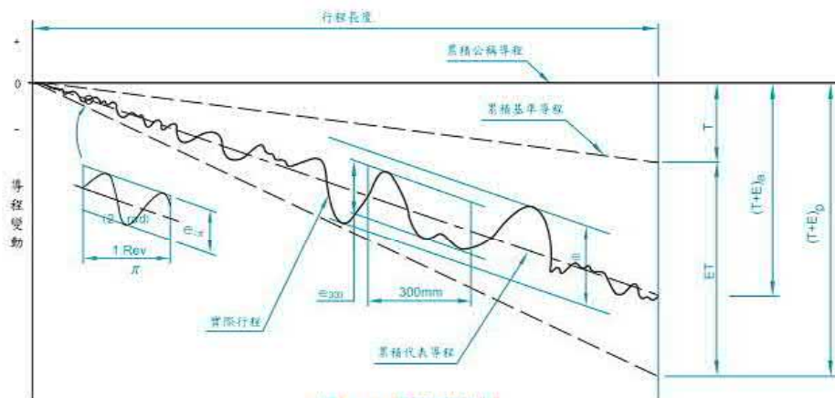
圖 4.1.1.1 導程量測曲線
