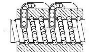
圖 4.3.1.2 外循環螺帽圖
