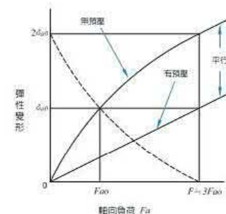
圖 4.4.1.5 彈性變形曲線
